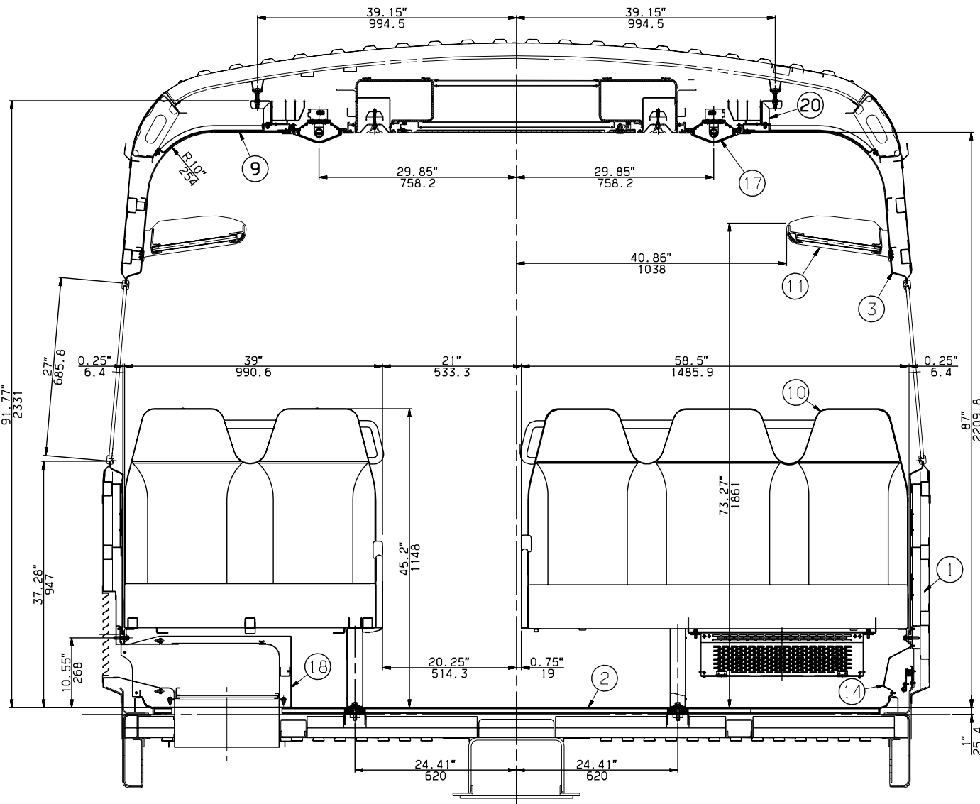
SECTION D-D
